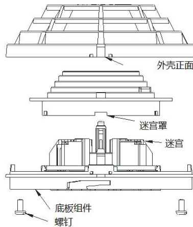
图 4. 产品清洁
