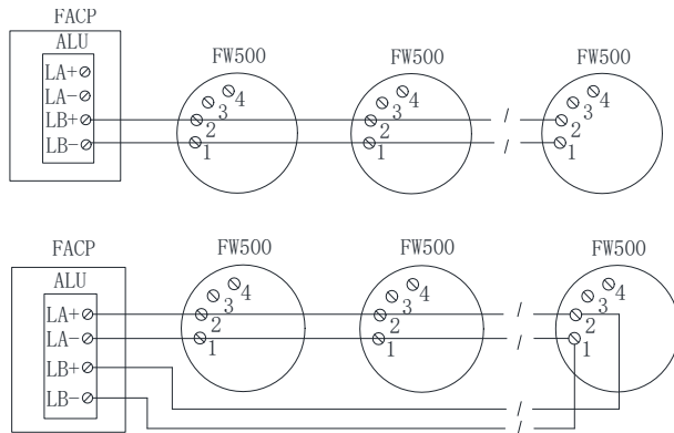
图 3. 产品接线
